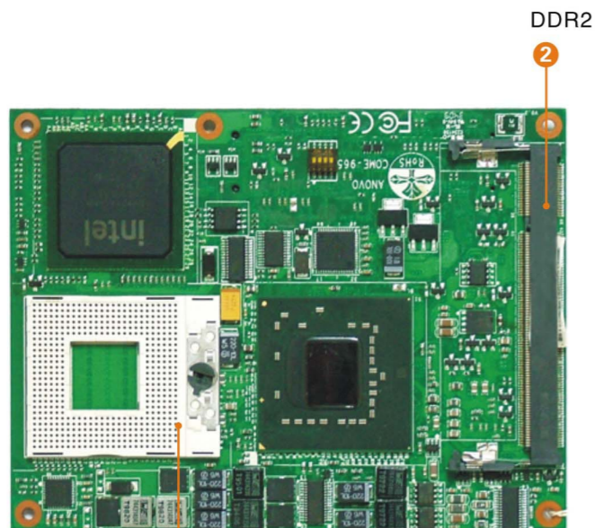
1 Socket 479
